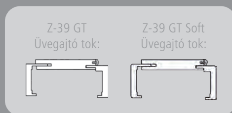
Tokkialakítás
