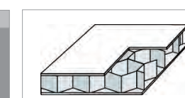
Papírrács térkitöltés
